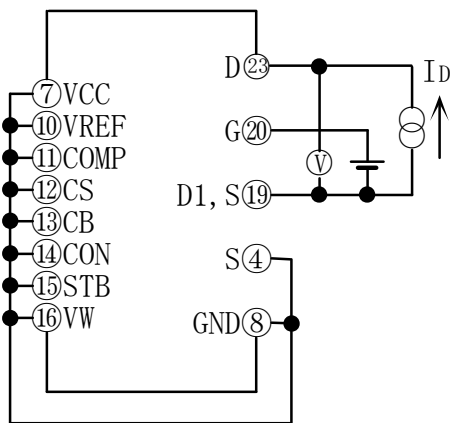
Fig.5 RDS(ON):Q2
