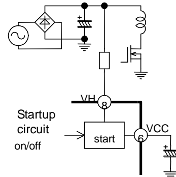
Fig.24 VH pin circuit (1)
