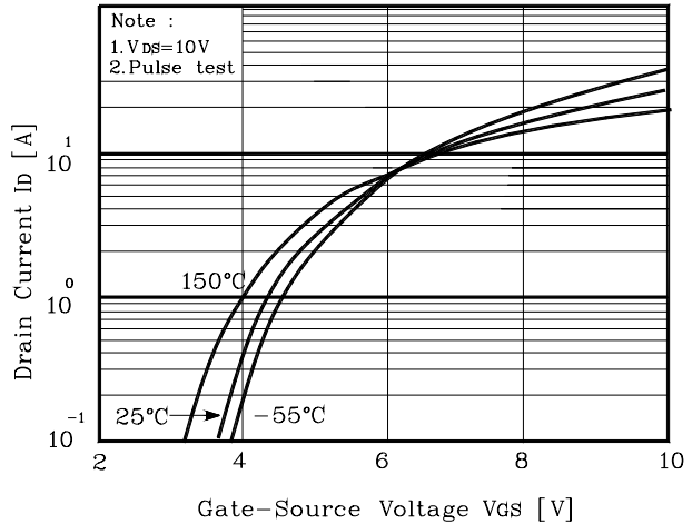
Fig. 2 I_D - V_{GS}
