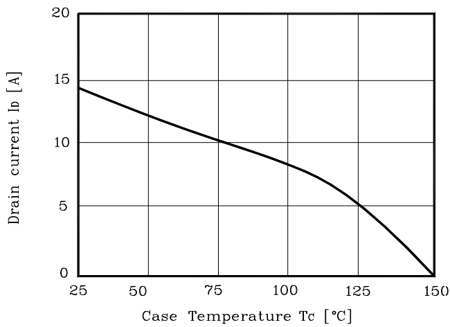
Fig. 9 I_D - T_C
