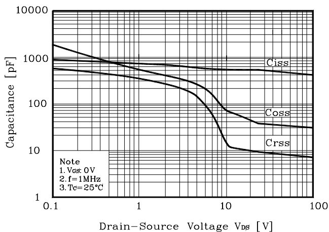
Fig. 5 Capacitance - V_{DS}
