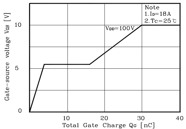
Fig. 6 V_{GS} - Q_G
