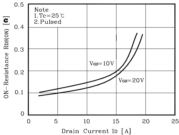
Fig. 3 R_{DS(on)} - I_D
