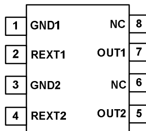
ESOP8
