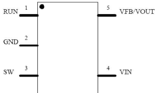
TSOT23-5
