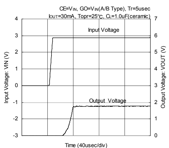
XC6217x182xx
