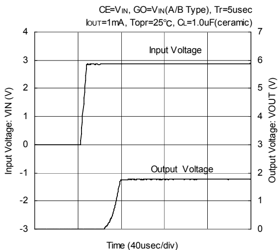
XC6217x182xx
