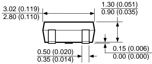
SOT-23-5 (M5)
