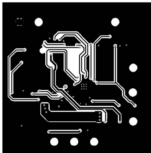
FIGURE 28. BOTTOM LAYER
