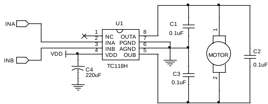
图 1：典型应用方案应用电路图
