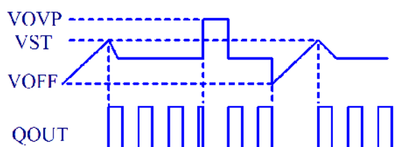
Fig6. UVLO
