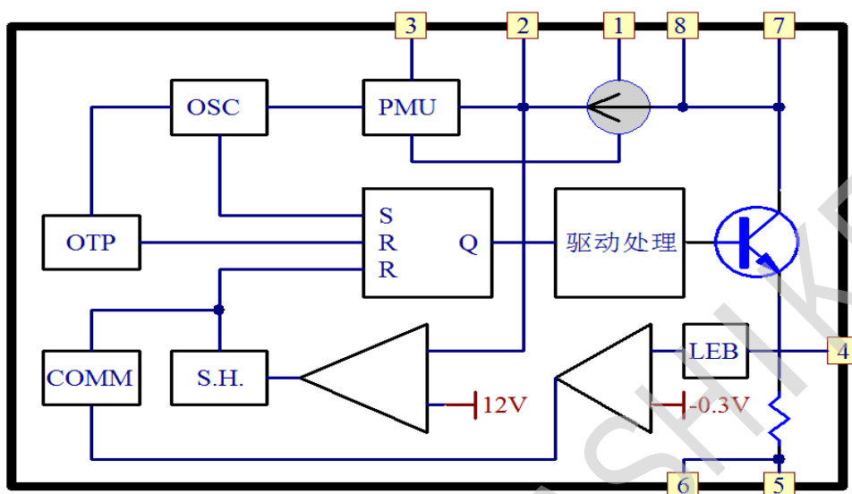
Fig2. 內部框圖
