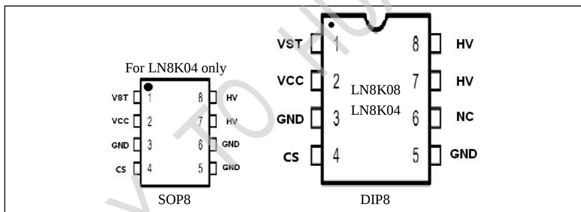
Fig3. 引腳定義
